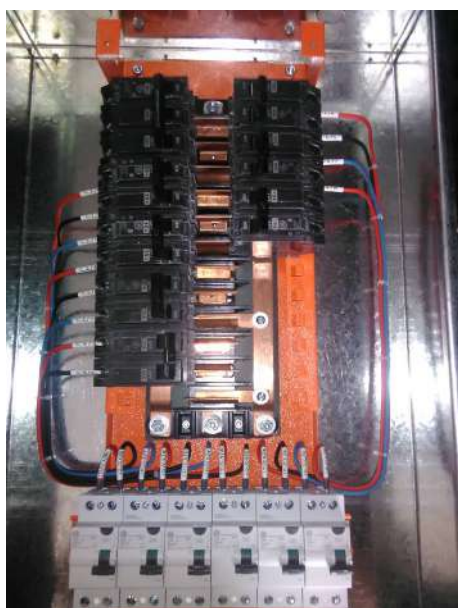
Diseño de Distribución (ITM + Diferencial): Tipo Empotrado,
