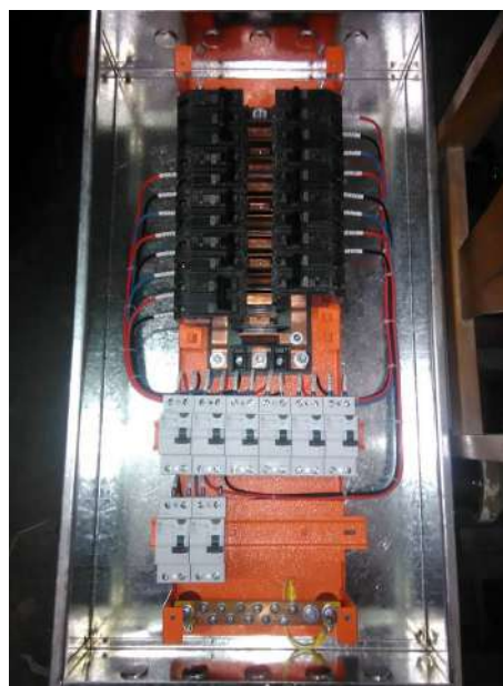
Diseño de Distribución (ITM + Diferencial): Tipo Empotrado,
